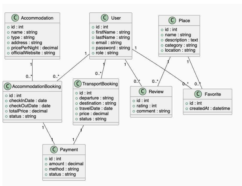
Figure 3.2 Diagramme de classe
