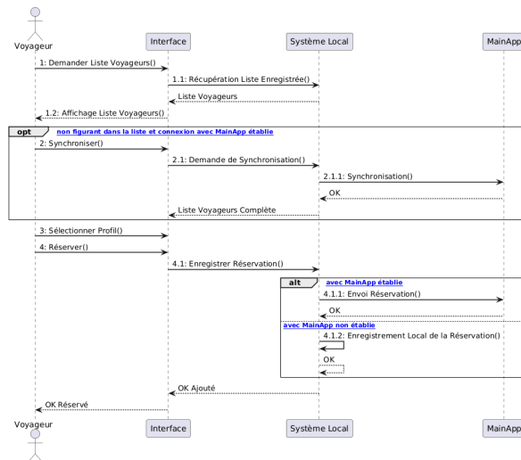
Figure 3.9 Diagramme de séquence-Réserve de transport
